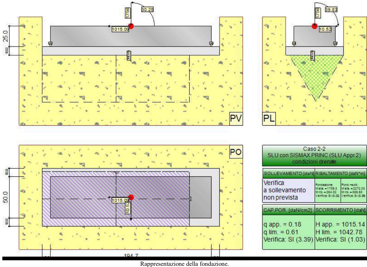
Rappresentazione della fondazione.
